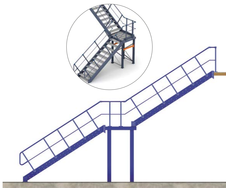
Schody s odpočívadlem (průběžné schody s odpočívadlem)
